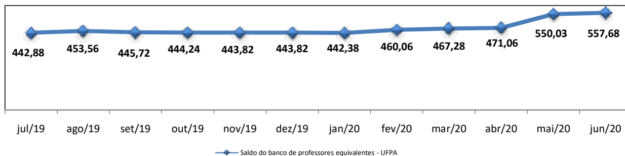
Saldo do banco de professores equivalentes - UFPA Julho/2019 a Junho/2020
